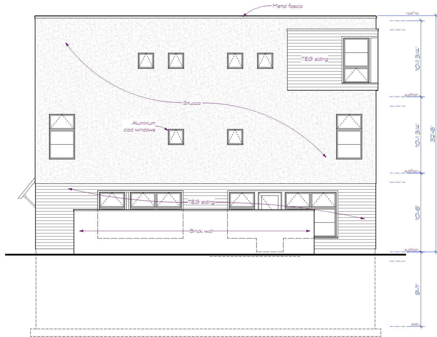
LEFT SIDE ELEVATION 4 SCALE: 1/8" = 1'-0"
