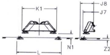
OUTRIGGER OPTION
